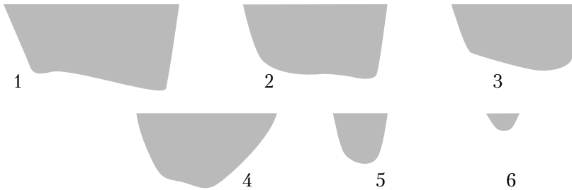
Схема 1. Профили поперечного сечения р.Лум (номера соответствуют номерам мест измерений в Таблице 1)
