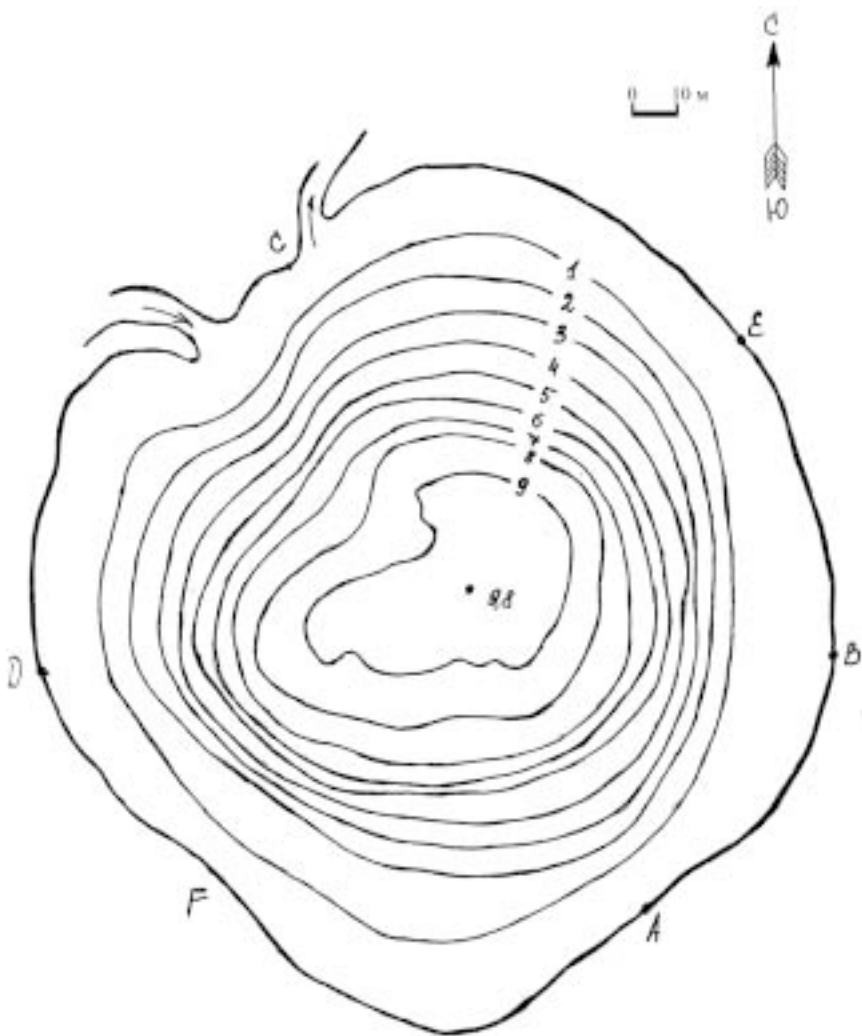
Рис. 2. Батиметрическая схема Никулятского озера. Выполнена М. Ершковой. 2007 год.
